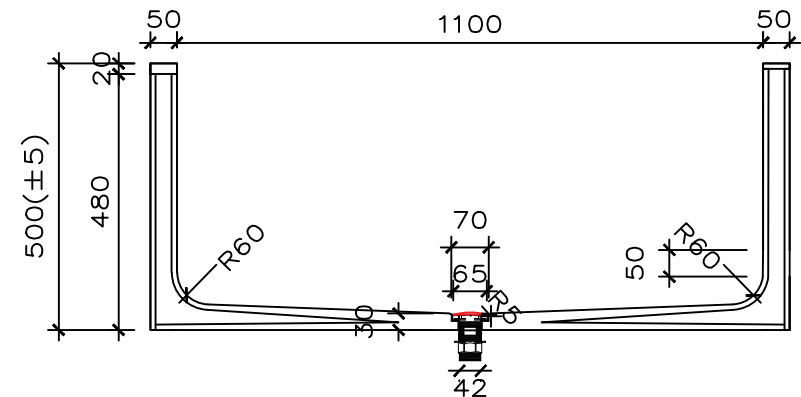
MẶT ĐỨNG
