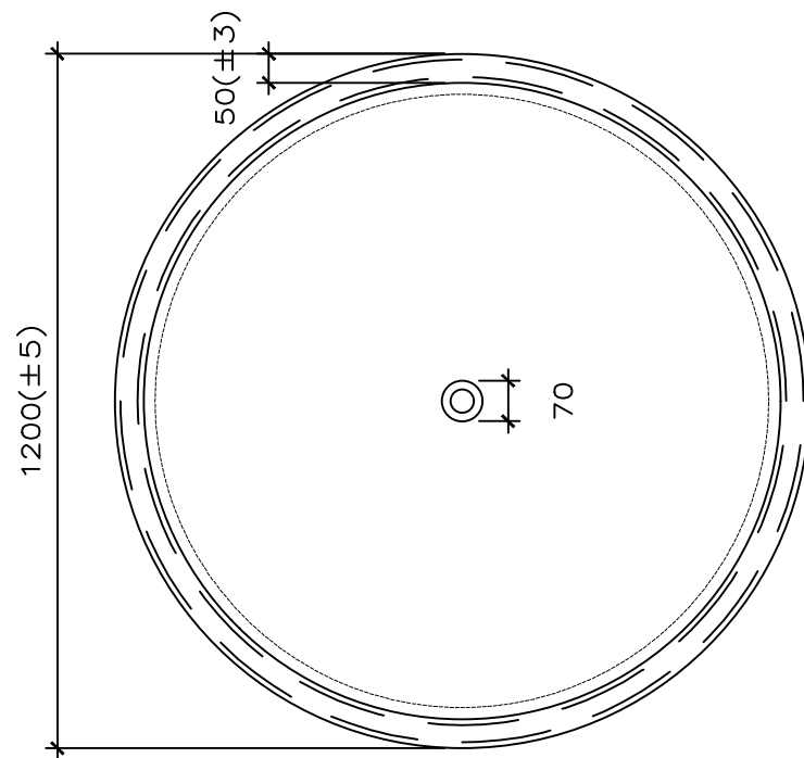
MẶT BẰNG
