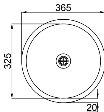
MẶT BẰNG
