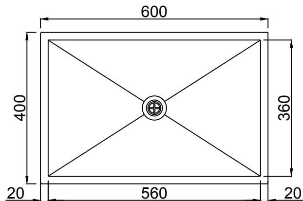
MẶT BẰNG
