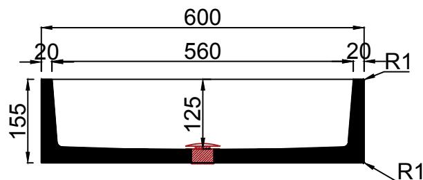
MẶT CẮT
