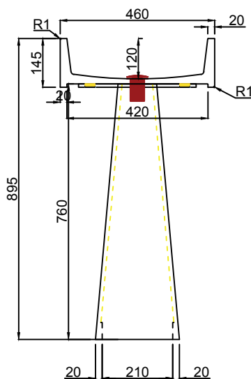
MẶT ĐỨNG
