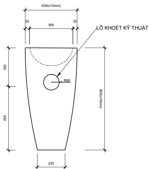
MẶT ĐỪNG
