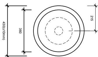
MẶT BẰNG
