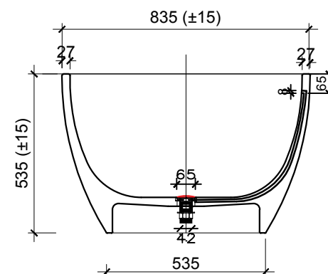
MẶT BÊN
