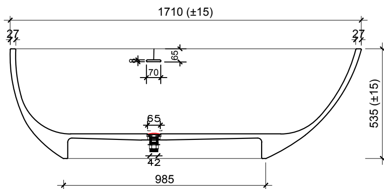
MẶT ĐỨNG
