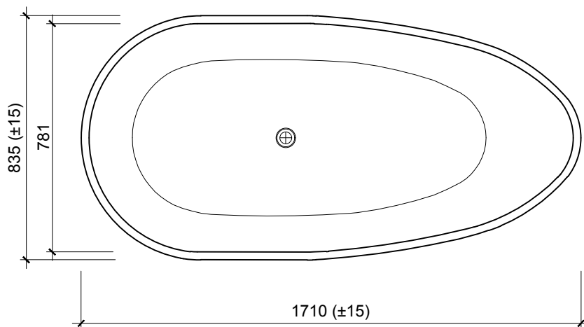
MẶT BẰNG
