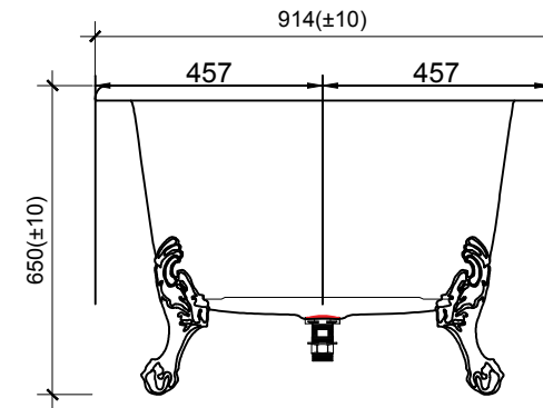
MẶT BÊN
