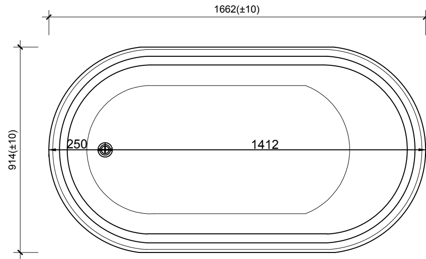
MẶT BẰNG
