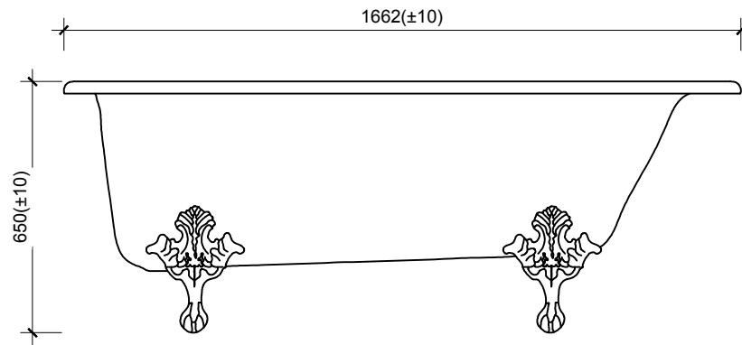
MẶT ĐỨNG
