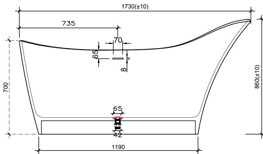
MẶT ĐỨNG
