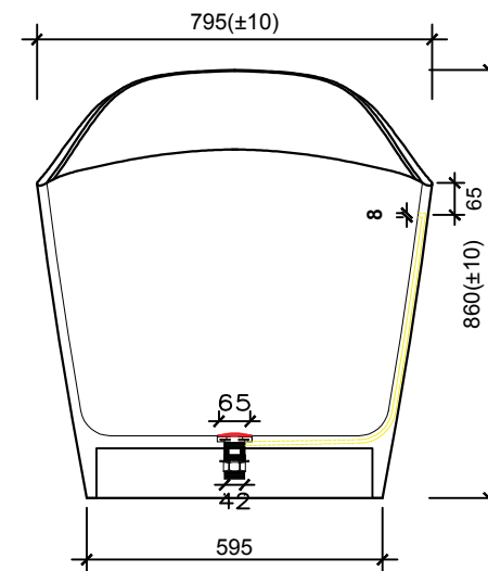
MẶT BÊN
