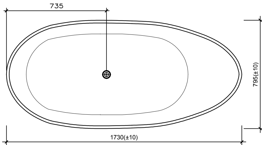
MẶT BẰNG
