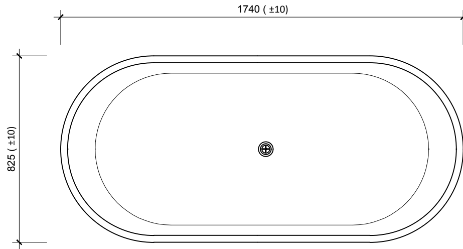
MẶT BẰNG
