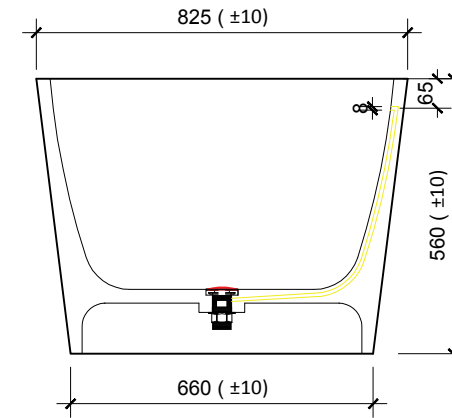
MẶT BÊN
